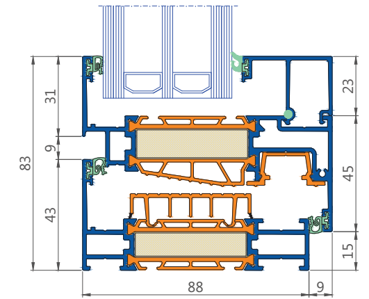
verticale doorsnede
